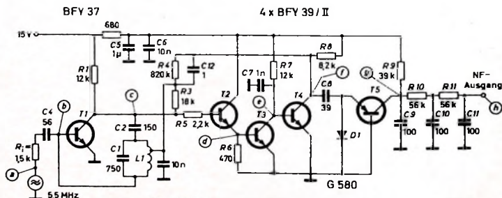
Bild 4. Gesamtschaltung des Ton-ZF-Teils
