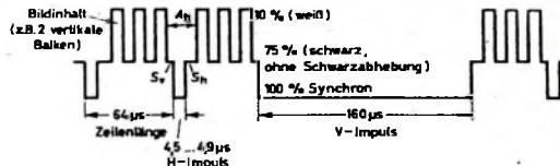
Bild 9. Normwerte der Synchron- und Austastimpulse; S v vordere Schwarzscher (1,3 1,8 µs), S h hintere Schwarzscher (5,1 bis 6,5 µs), A h Horizontalaustastung (11,8 12,3 µs); Vertikal-austastung 1,125...1,4 ms (18 bis 22 Zeilen)
