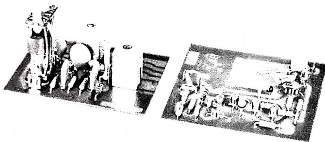
Bild 2. Versuchsaufbau der neuen Schaltung; links: Standardschaltung mit Verhältnisdiskriminator, rechts: neue Schaltung (integrierbar)
