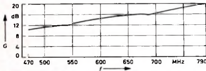
Gewinn G der 40-Elemente-UHF-Superbreitbandantenne (VEB Antennenwerke Bad Blankenburg)
