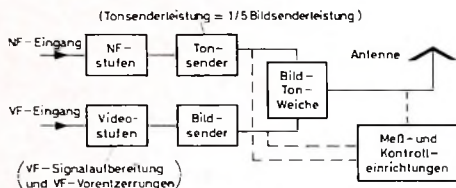
Bild 129. Blockbild eines Fernsehsenders
