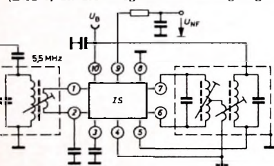
Bild 1. Die übliche Schaltung eines Fernseh-Ton-ZF-Verstärkers für 5,5 MHz in integrierter Schaltung (IS integrierter Schaltkreis)
