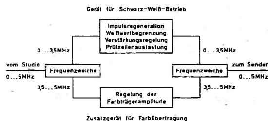
Bild 134. Fernsehseingangsverstärker für Farbübertragungen (Regeneration und automatische Verstärkungsregelung)
