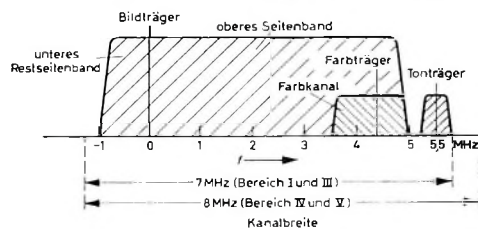
Bild 131. Spektrale Verteilung der Bild-, Ton- und Farbinformation im hochfrequenten Fernsehsignal
