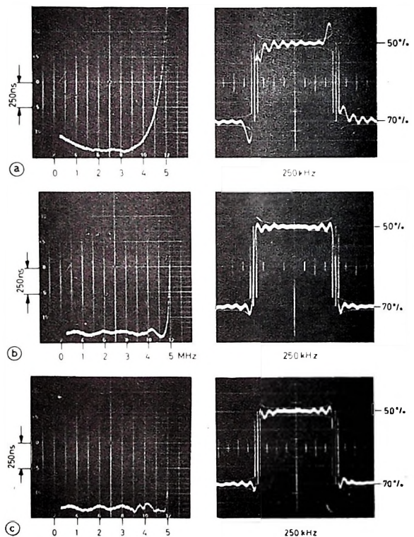
Bild 138. Laufzeitkurve und 250-kHz-Rechteckspannung, gemessen über Sender und Empfänger; a) ohne Phasenzerrter, b) mit Schwarz-Weiß-Entzerrung, c) mit Schwarz-Weiß-Entzerrung und Farbkanalentzerrer
