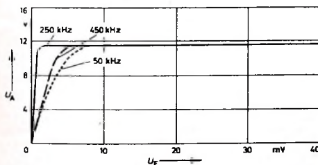
Bild 6. Begrenzungskennlinien; U_E = Spannung am Punkt a, U_A = ZF-Ausgangsspannung am Kollektor von T4 (Punkt f im Bild 4)
