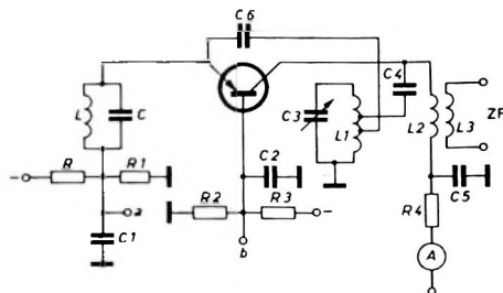
Bild 81. Messungen an einem Transistoroszillator
