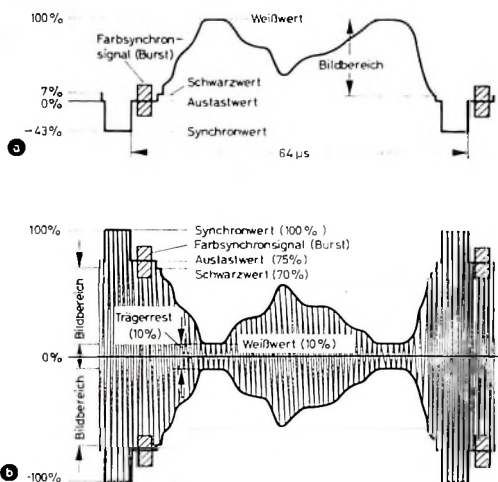
Bild 130. a) Videosignal am Sendereingang, b) hochfrequentes Fernsehsignal am Senderausgang und an der Antenne
