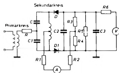
Bild 82. Messungen an einem Ratiodektor
